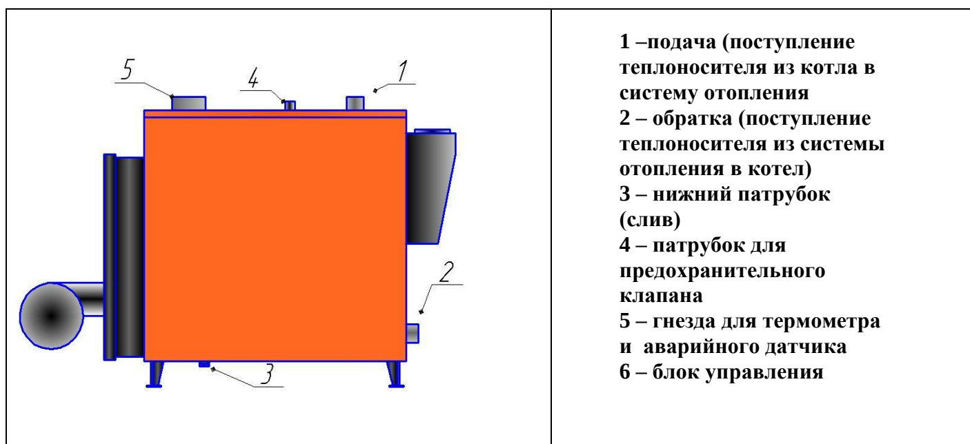
Рис.1 Внешний вид котла 41 кВт
